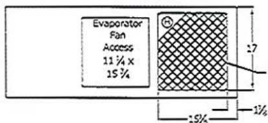
VIEW A-A
